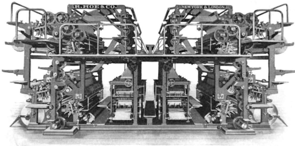
OCTUPLE PRESS
