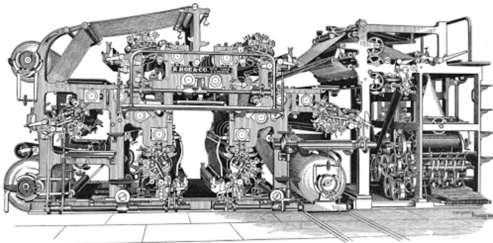
SEXTUPLE PRESS
