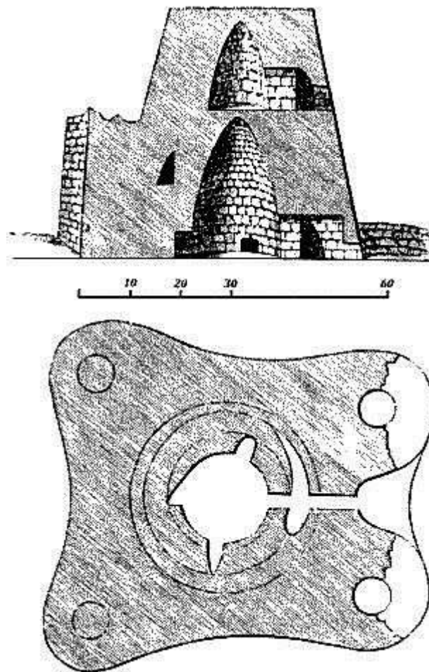
187. Nurhag of Santa Barbara. From De la Marmora.
