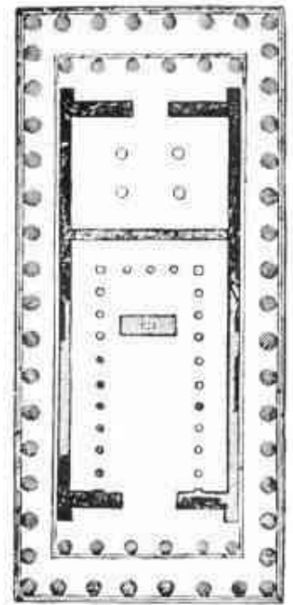
PARTHENON. OCTO- STYLE-PERIPTERAL
