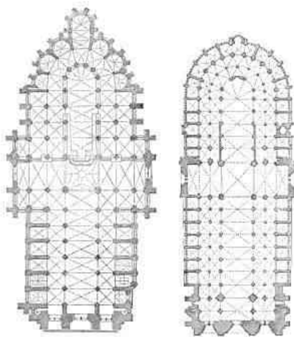
PLAN OF AMIENS
