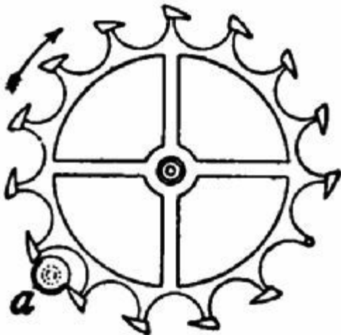
FIG. 204.—"Cylinder" watch escapement.
