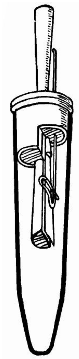
FIG. 144.—A reed pipe.
