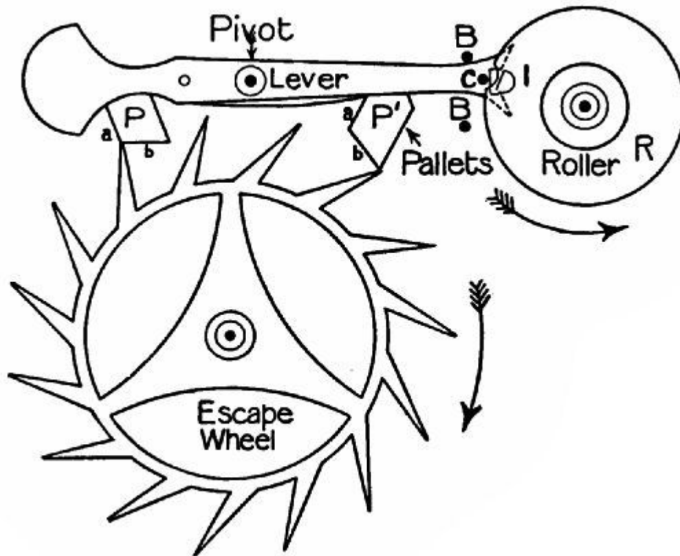
FIG. 205.—"Lever" watch escapement.
