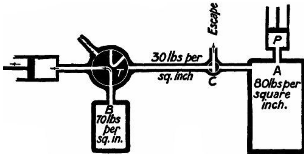
FIG. 89.—Brake "on."
