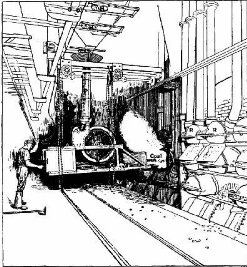
FIG. 198.—De Brouwer automatic retort charger.
