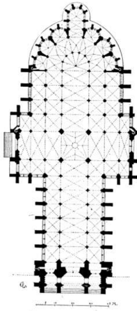
47. AMIENS CATHEDRAL. PLAN
