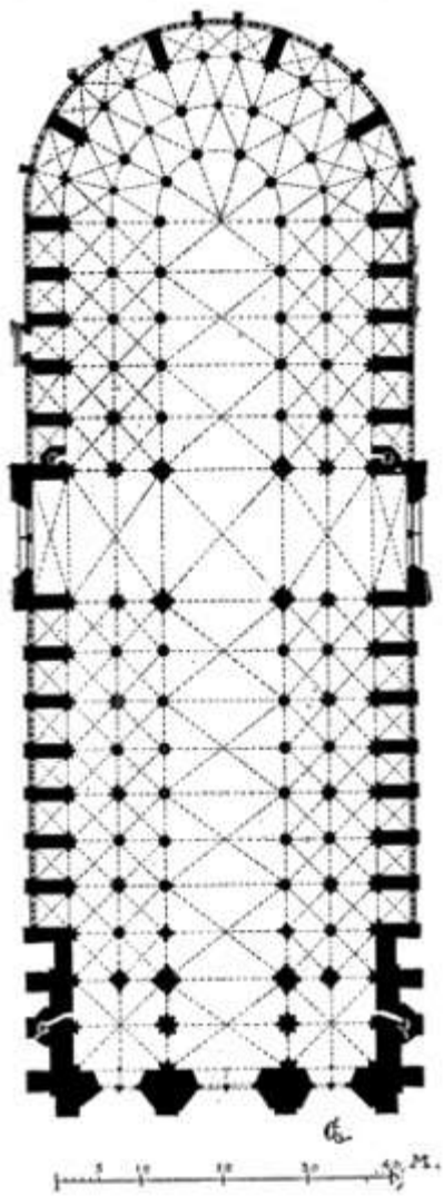
37. NOTRE DAME DE PARIS. PLAN
