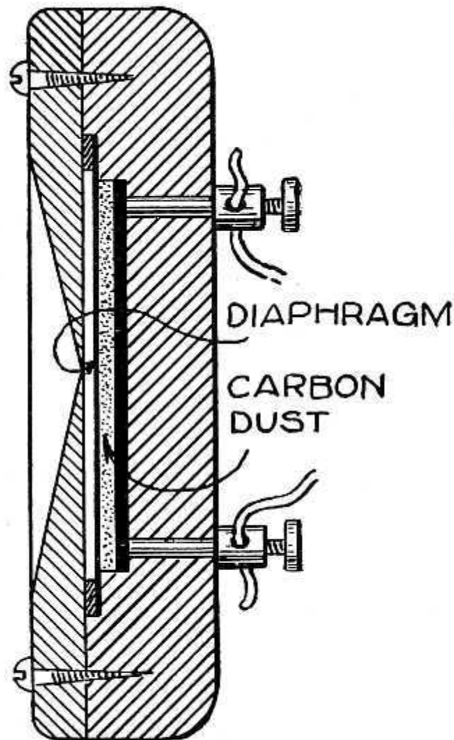
FIG. 71—CARBON-DUST TRANSMITTER
