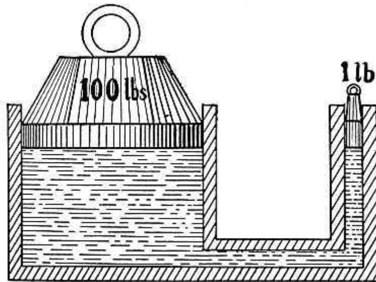
FIG. 8—A SIMPLE HYDRAULIC PRESS
