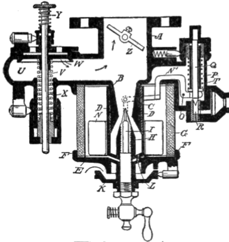
Fig. 31. Carbureter.
