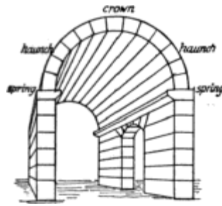
FIG. 46.—BARREL VAULT.
