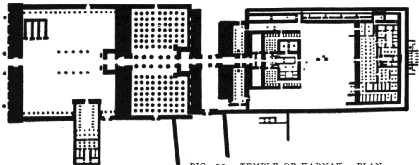
FIG. II.—TEMPLE OF KARNAK. PLAN.
